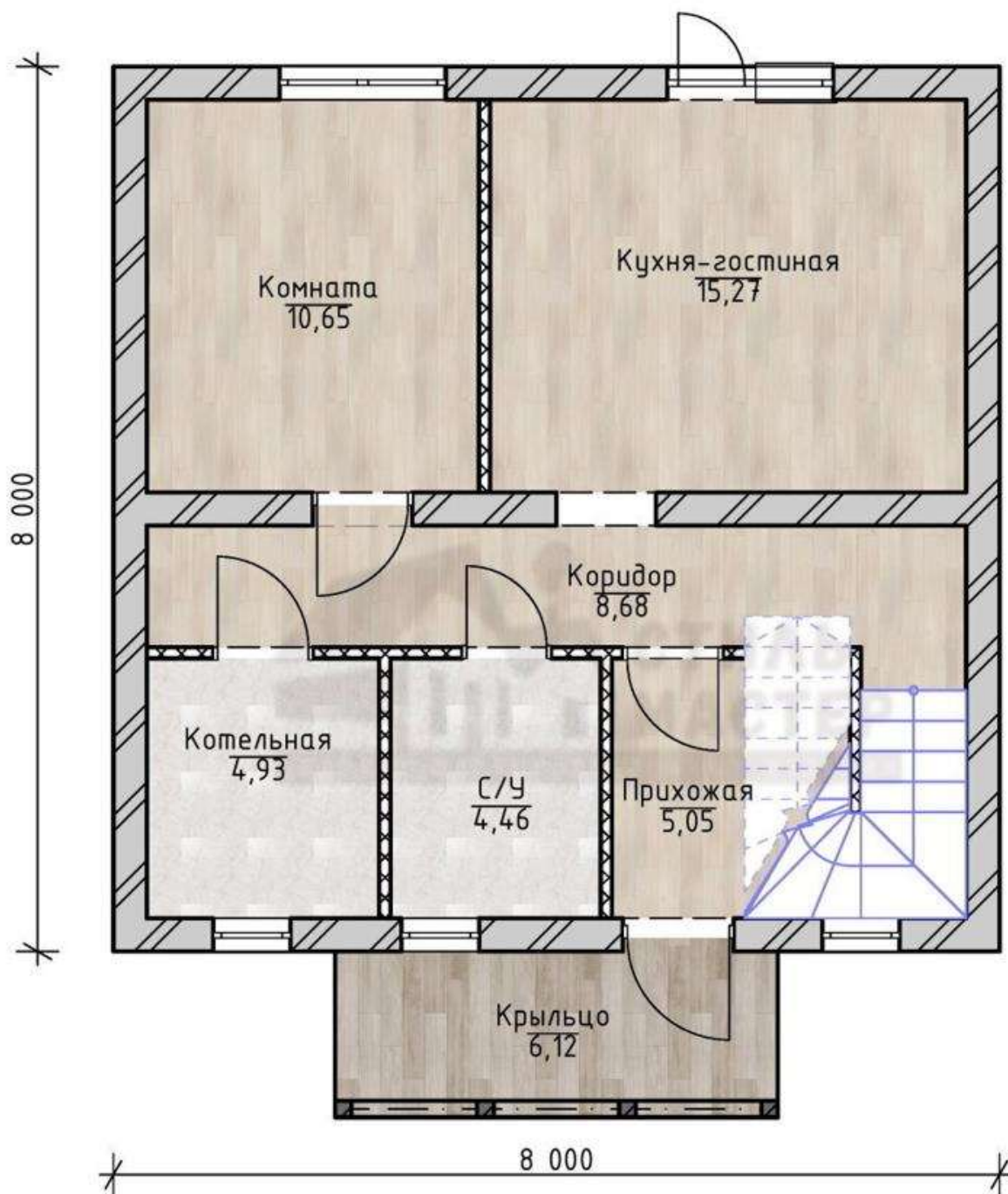
План 1 этажа
